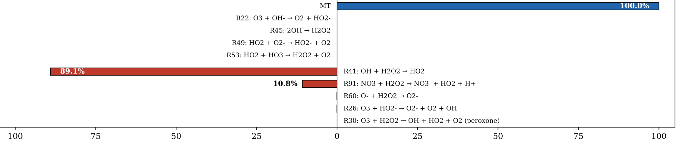
(d) H 2 O 2 (Σsrc = 4.35e-09 M/s)
